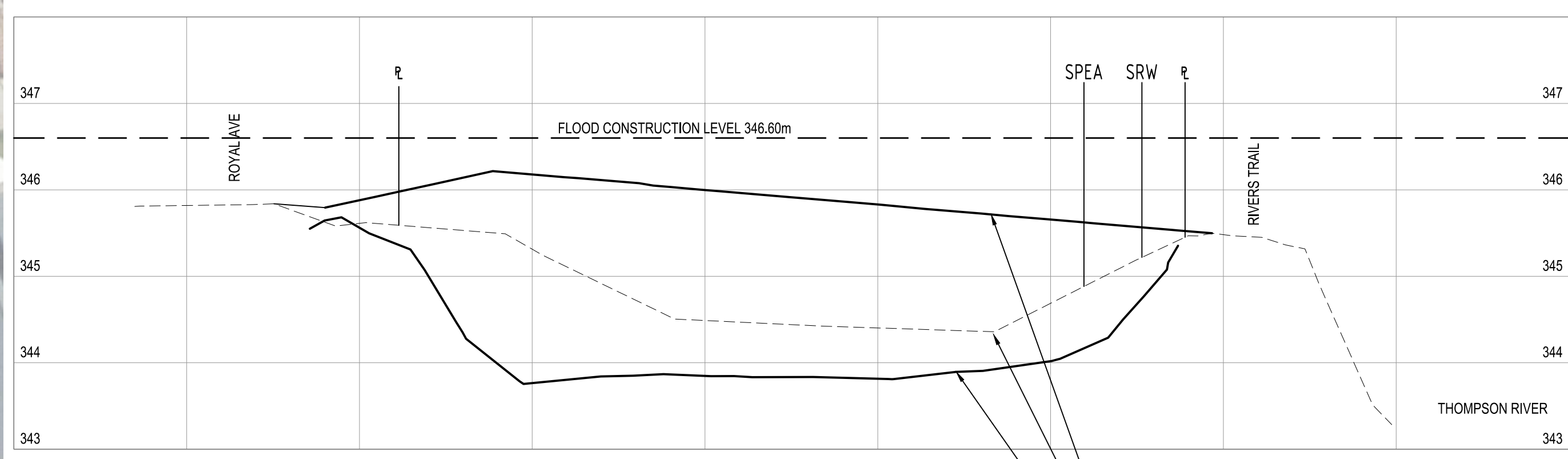
SECTION B - B SCALE: 1:250 H 1:50 V
