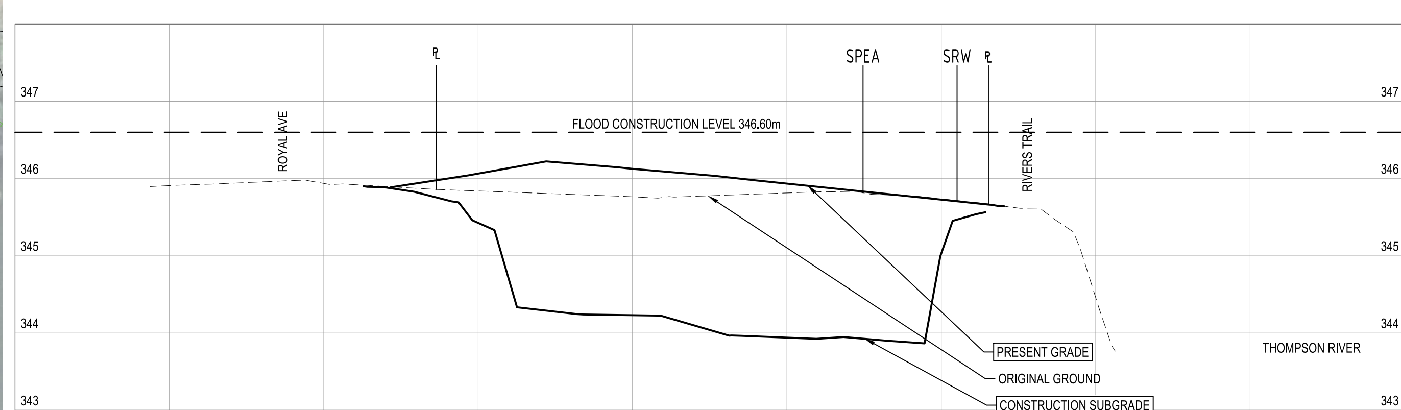
SECTION C - C SCALE: 1:250 H 1:50 V
