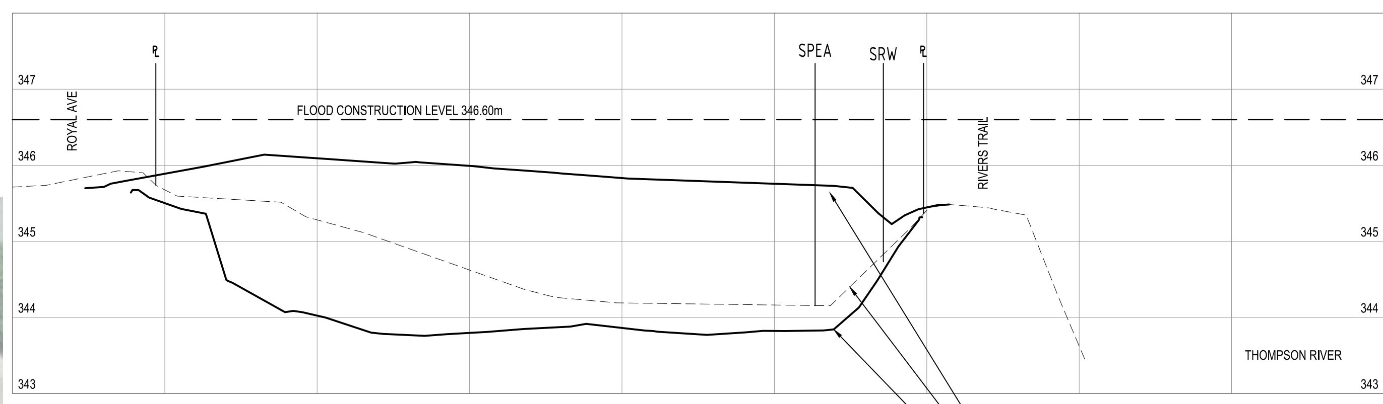
SECTION A - A SCALE: 1:250 H 1:50 V
