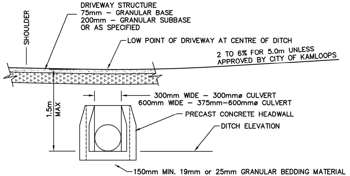
ELEVATION
